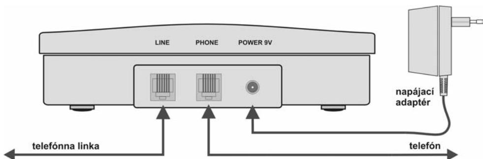
obr. 1: Zapojenie terminálu
